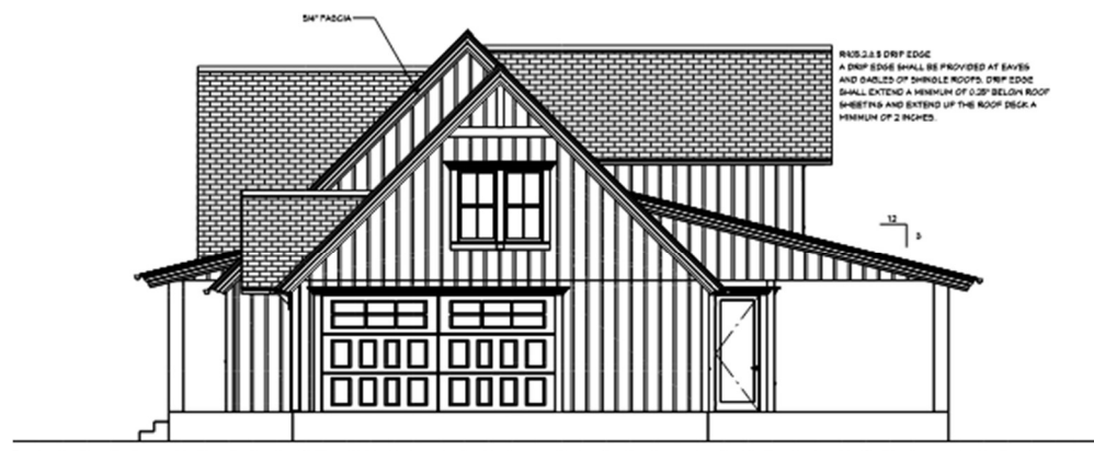
RIGHT ELEVATION
